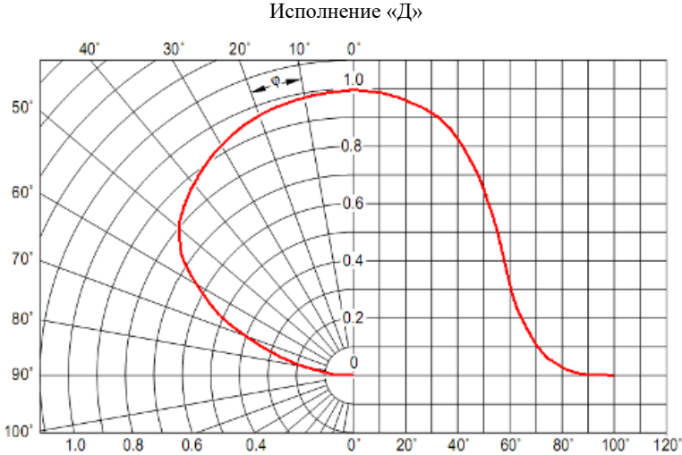
Рисунок 4 Тип КСС
