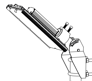
Поворотная консоль
