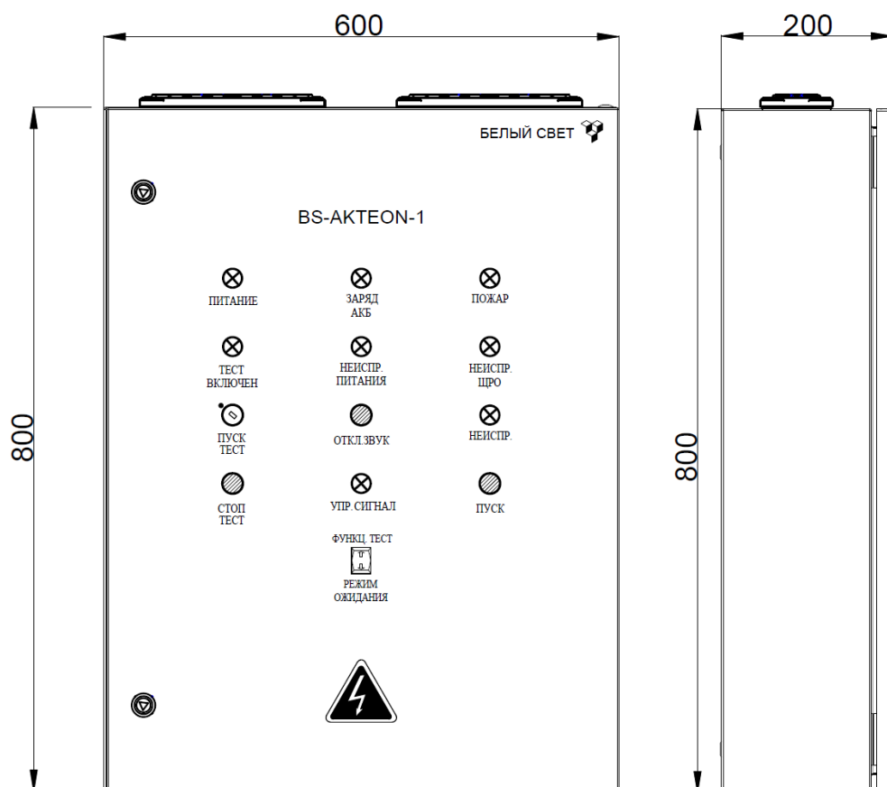
Рис. №1 Габаритный чертёж.
