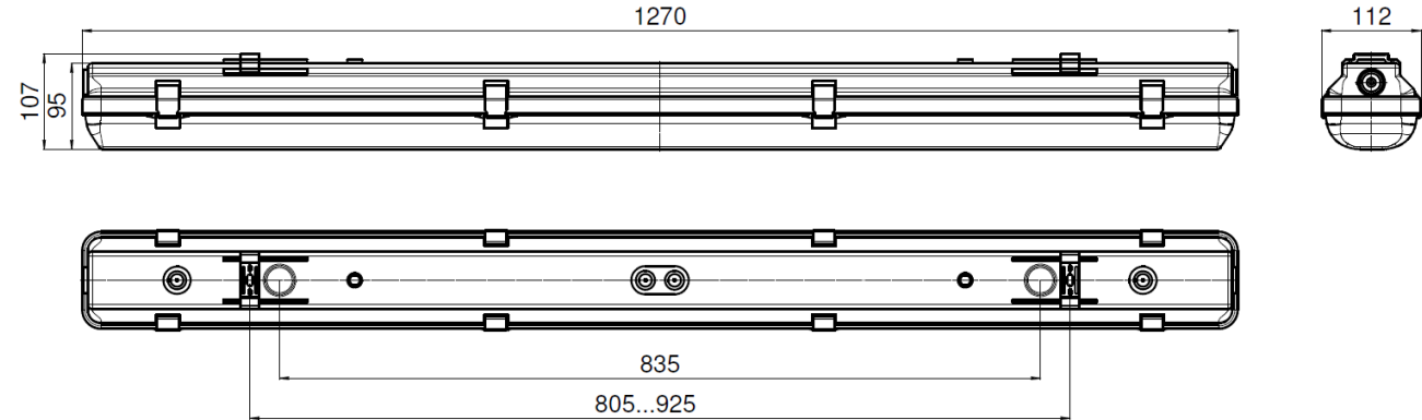
Рис. №5 Габаритный чертёж
