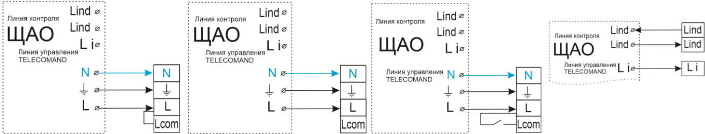
Рис. №1.1, 1.2, 1.3, 1.4 Схема подключения к групповой цепи питания и управления.
