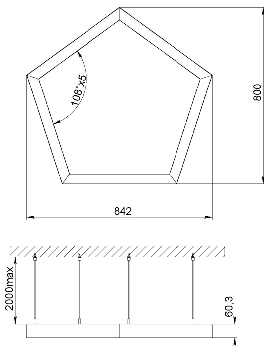
Рис.1 Габаритный чертеж.
