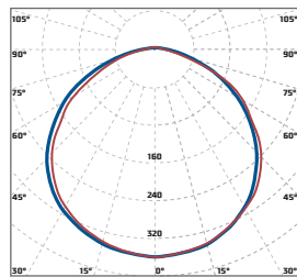
«Diora Unit Дв» косинусная КСС 120°
