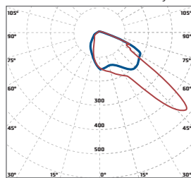
«Diora Unit Cross» асимметричная КСС 90°x20°
