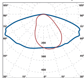
«Diora Unit PRO Ш» широкая боковая КСС 150°x75°
