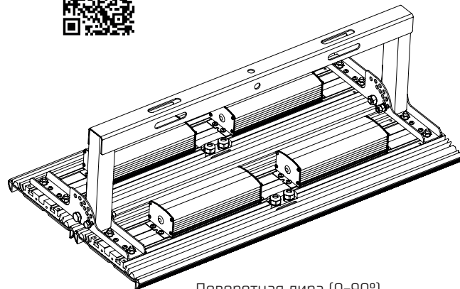
Поворотная лира (0-90°)
