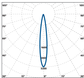
«Diora Unit K14» концентрированная КСС 14°
