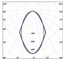
«Diora Unit K60» глубокая КСС 60°
