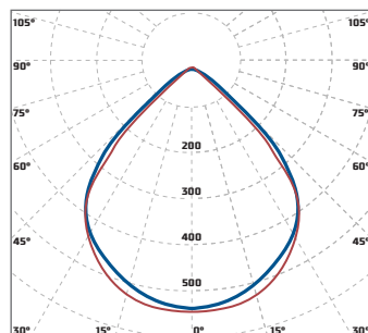
«Diara Unit Г90» глубокая КСС 90°
