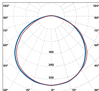
«Diara Unit Д» косинусная КСС 120°
