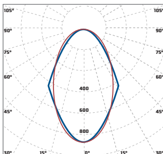
«Diara Unit K60» глубокая КСС 60°
