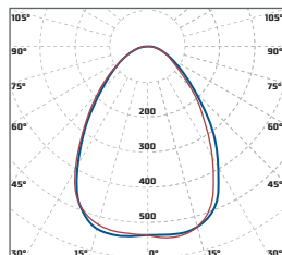
«Diora Quadro Track Г80» глубокая КСС 80°
