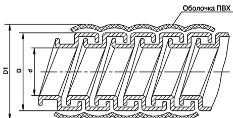
Рисунок 2 – Металлорукава РЗ-ЦП
