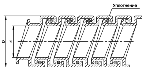
Рисунок 1 – Металлорукава РЗ-ЦХ
