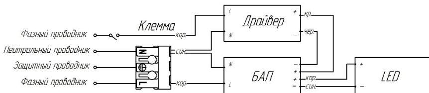
Рис.5 Принципиальная схема подключения с блоком аварийного питания.
