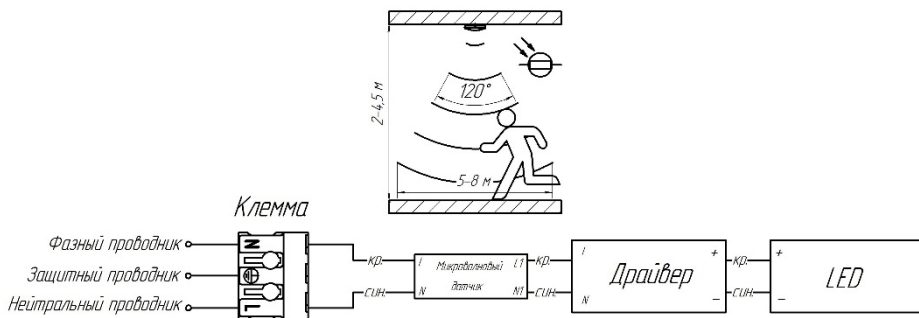
Рис.4 Принципиальная схема подключения с микроволновым датчиком.
