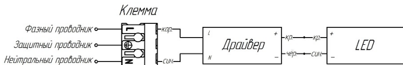
Рис.3 Принципиальная схема подключения.
