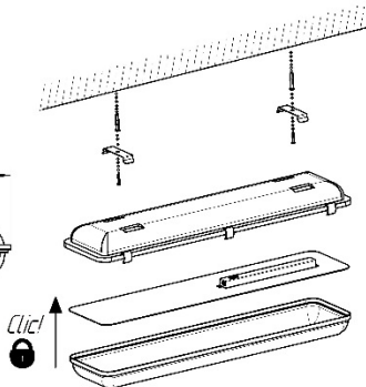
Рис.2 Монтажная схема.
