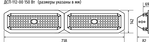
ДСП-112-00 150 Вт (размеры указаны в мм)
