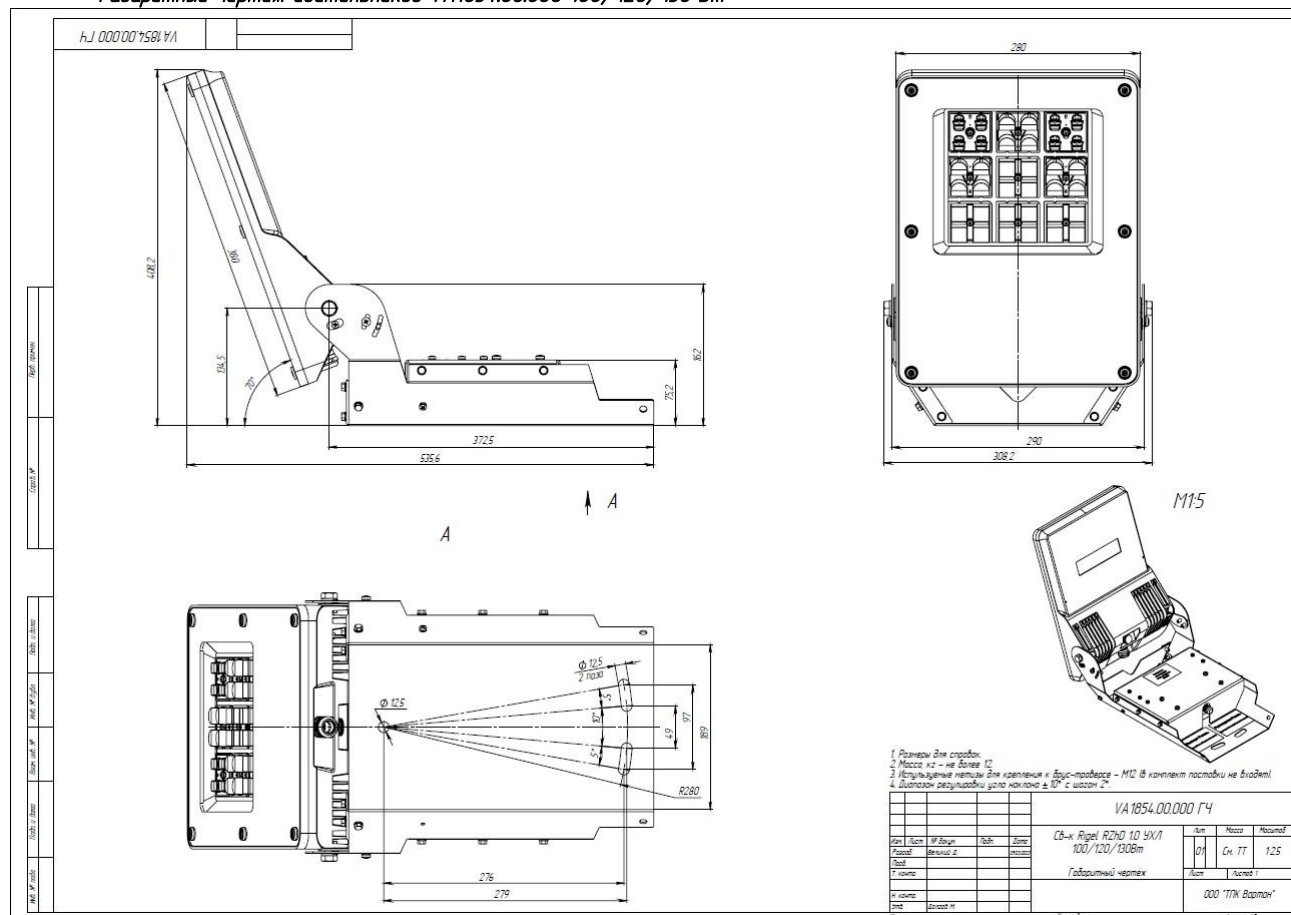
Габаритный чертёж светильников VA1854.00.000 100/120/130 Вт
