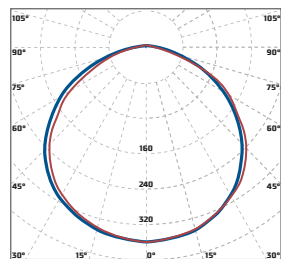
«Diora Unit Д» косинусная КСС 120°
