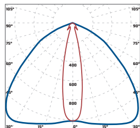
«Diora Unit Store» специальная КСС 105x25°
