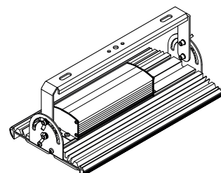
Поворотная лира [0-180°]
