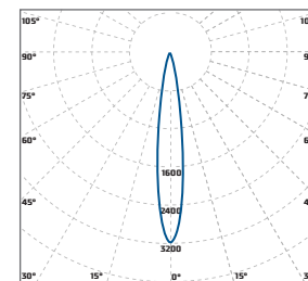
«Diora Unit К14» концентрированная КСС 14°
