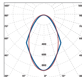
«Diora Unit К60» глубокая КСС 60°
