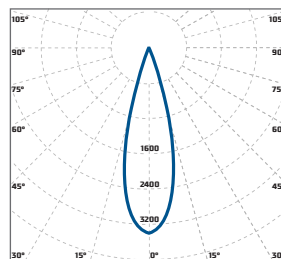
«Diora Unit К30» концентрированная КСС 30°
