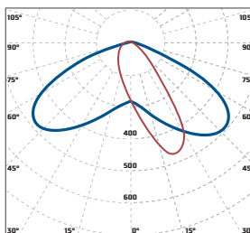
«Diora Unit PRO Ш1» широкая боковая КСС 130°x40°
