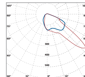
«Diora Unit Cross» асимметричная КСС 90x20°
