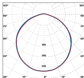
«Diora Unit Frost Д» косинусная КСС 115°
