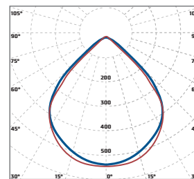
«Diora Unit Г90» глубокая КСС 90°
