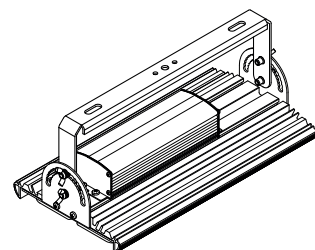
Поворотная лира [0-180°]
