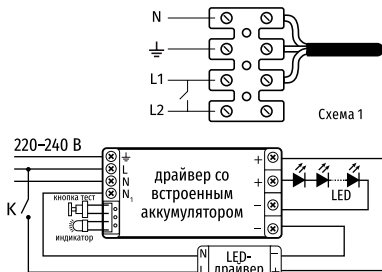
Схема подключения БАП в светильнике ДВО-15-А
