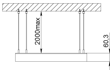
Рис.1 Габаритный чертеж.
