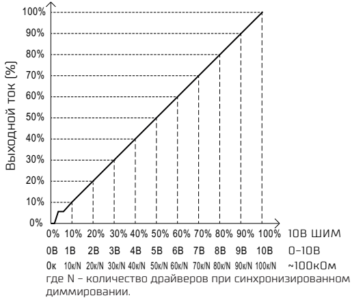
Б) График зависимости при регулировке «DA»:
