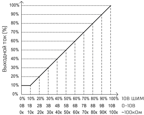
А) График зависимости при регулировке «i»:
