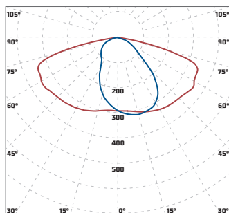
«Diora Skat ШБ4» широкая боковая КСС 150°x70°
