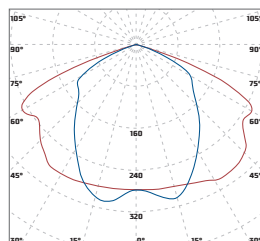
«Diora Meduza ЛО» полуширокая осевая КСС 140°x95°
