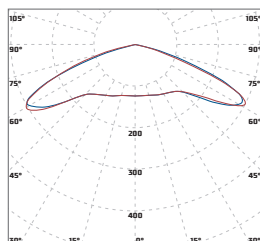
«Diora Meduza ШК» широкая круглосимметричная КСС 140°
