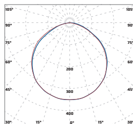
«Diora Meduza Д прозрачный» косинусная КСС 110°
