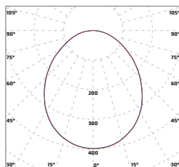
«Diora Meduza Д opal» косинусная КСС 100°
