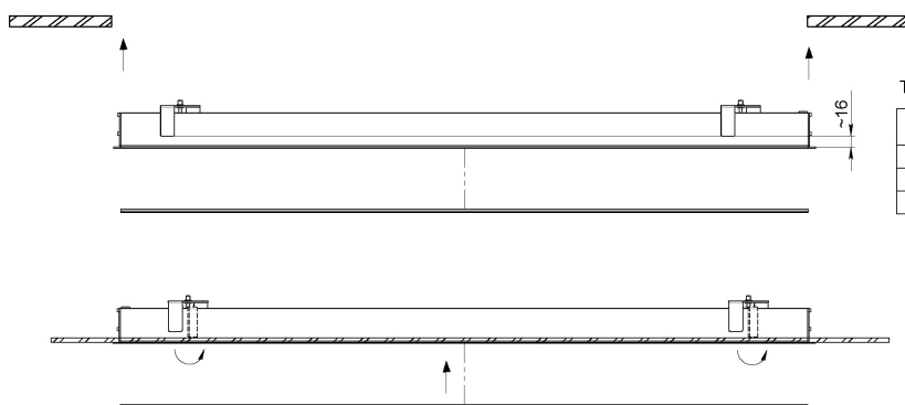
Рис. 2. Монтажный чертеж.
