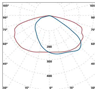
«Diora Skat ШБ3» широкая боковая КСС 150°x90°
