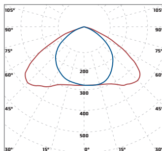
«Diora Skat ШО» широкая осевая КСС 125°x105°
