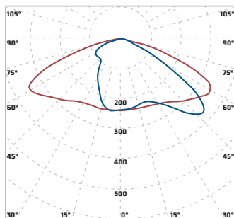
«Diora Skat ШБ1» широкая боковая КСС 140°x80°
