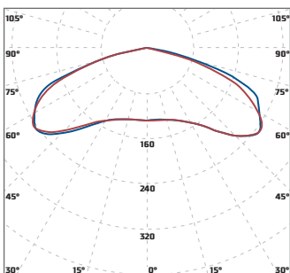
«Diora Skat ШК» – широкая круглосимметричная КСС 145°
