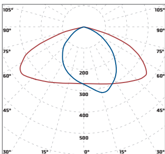
«Diora Skat ШБ2» широкая боковая КСС 140°x90°
