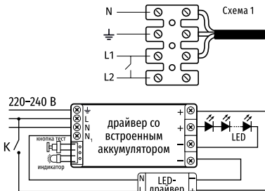
Схема подключения БАП в светильнике ДВО-18-A
