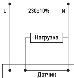
Рисунок 5. Схема подключения датчиков ДД 201B
