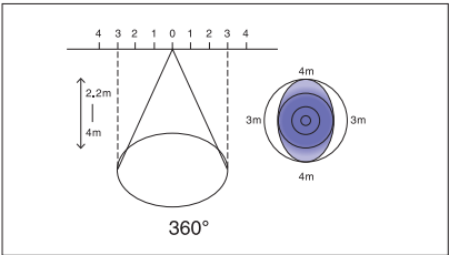
Рисунок 2. Диаграмма направленности ДД 20B5
