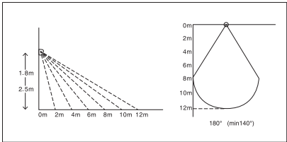
Рисунок 1. Диаграмма направленности ДД 08 / ДД 09
