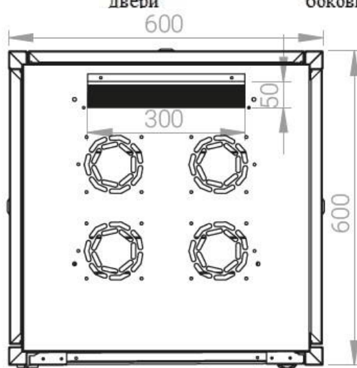
вид спереди без двери
