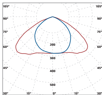
«Diora Skat ШО» широкая осевая КСС 125°x105°
