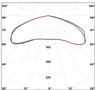
«Diora Skat ШК» – широкая круглосимметричная КСС 145°
