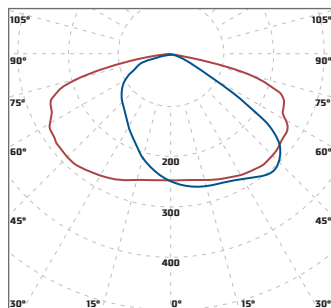
«Diora Skat ШБ3» широкая боковая КСС 150°x90°
