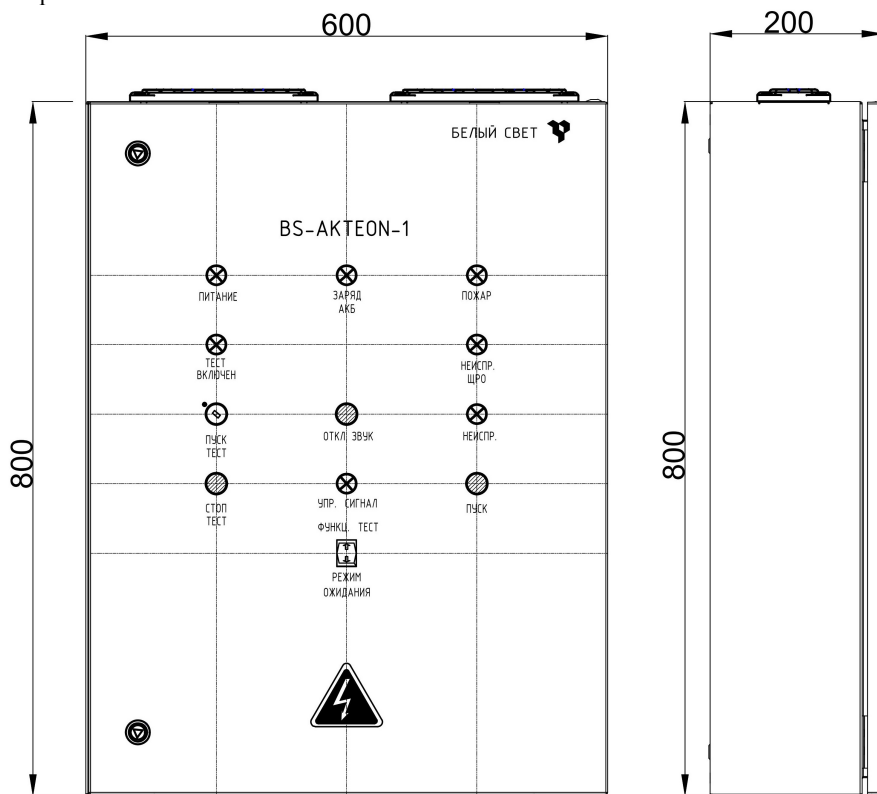
Рис. №1 Габаритный чертёж.
