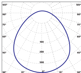
«Diora Office IP65 prism » косинусная КСС 90°
