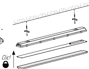
Рис.2 Монтажная схема.
