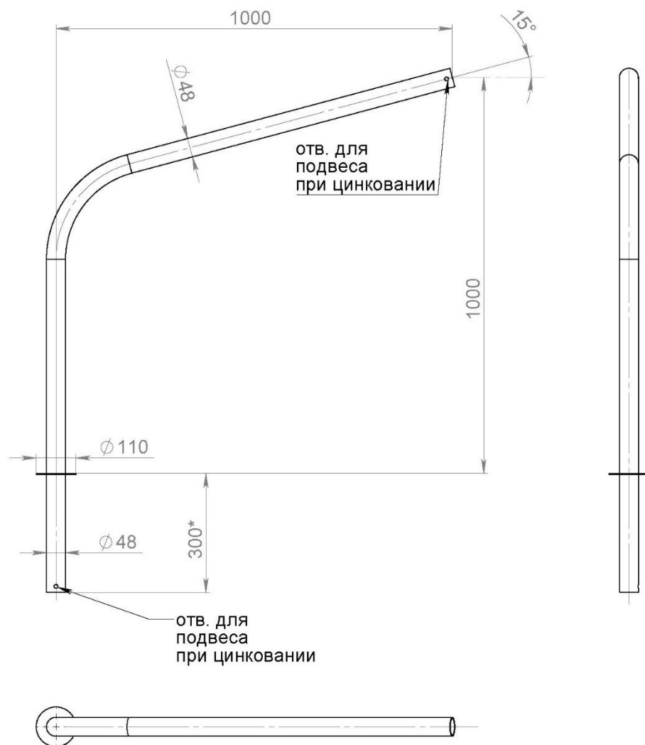
Рис.1 - Габаритные и присоединительные размеры
