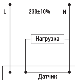
Рисунок 5. Схема подключения датчиков ДД 201B
