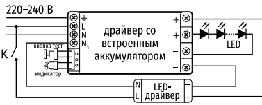
Схема подключения БАП в светильнике ДВО-14-А
