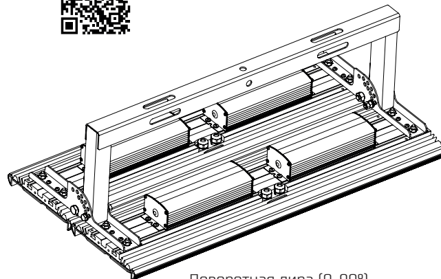
Поворотная лира (0-90°)
