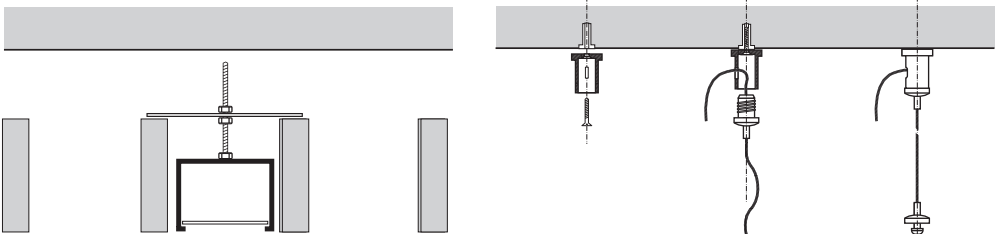
Рис.3 Схема монтажа светильника в реечный потолок при помощи комплекта креплений ШК 4895205052291
