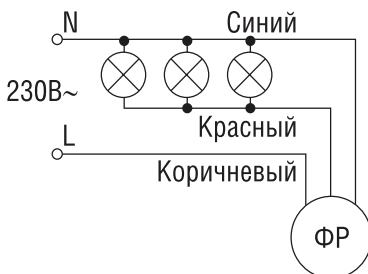
Рисунок 1. Схема подключения фотореле
