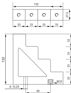
Рис. 2 - Изолятор «Лесенка» 450 А 9 кВ
