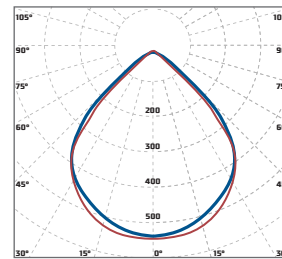
«Diora Unit Г90» глубокая КСС 90°
