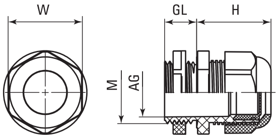
Рисунок 1. Основные размеры сальников.
