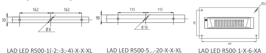
Рис. 1. Крепежные отверстия
