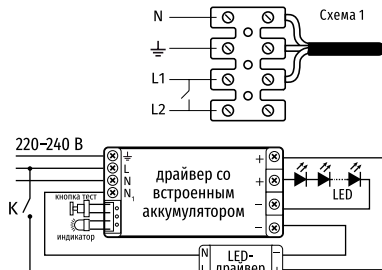
Схема подключения БАП в светильнике ДВО-А
